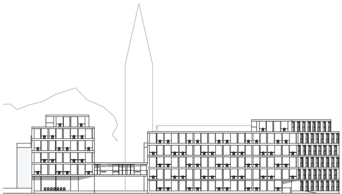
SÜD-ANSICHT 1 zu 200
